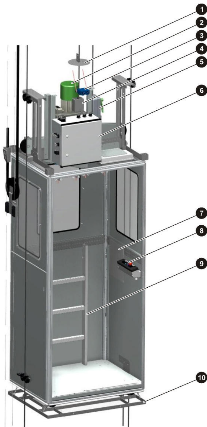
Bild 2: Aufstiegshilfe (innen)
